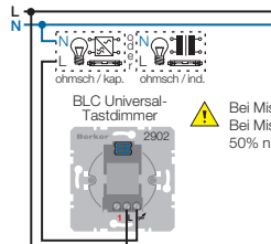
Grundschaltung
