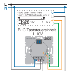
Grundschaltung
