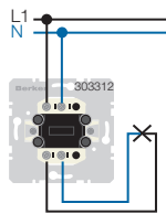
Ausschaltung 2-polig
