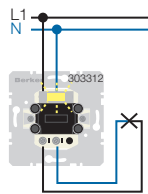
Ausschaltung 2-polig Dauerbeleuchtet (Glimmaggregat 160002 leuchtet immer)
