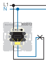
Ausschaltung 2-polig Kontroll (Glimmaggregat 160002 leuchtet bei "Ein")
