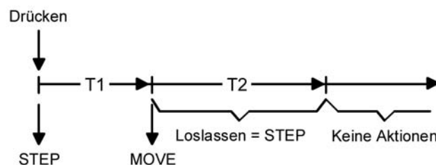
Bild 12: Bedienkonzept "Kurz-Lang-Kurz"
