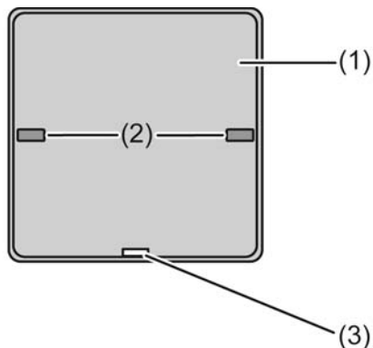
Bild 1: Geräteaufbau Tastsensor Komfort 1fach
