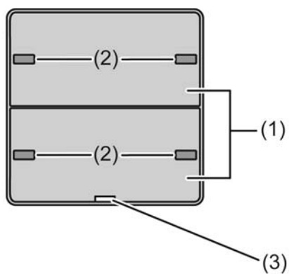
Bild 2: Geräteaufbau Tastsensor Komfort 2fach
