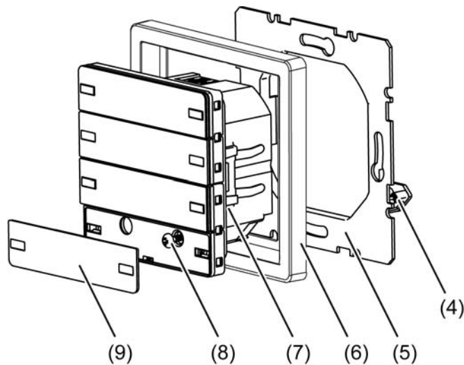
Bild 5: Gerätemontage am Beispiel eines Tastsensors Komfort 4fach
