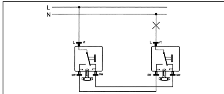
Anschlussbeispiel
