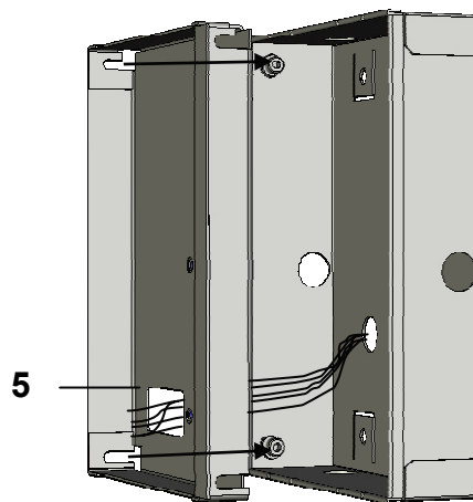
Einbaurahmen
