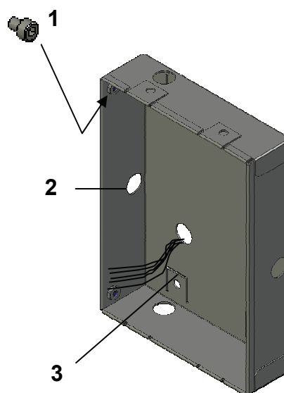
UP- Einbaugehäuse
