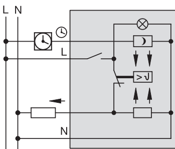
Raumtemperaturregler-Einsatz mit Schalter Art.-Nr. 5363..
