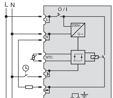
Fußbodentemperaturregler-Einsatz mit Schalter Art.-Nr. 537100
