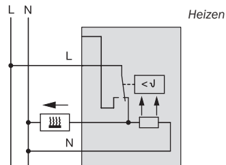
Raumtemperaturregler-Einsatz mit Wechselkontakt Art.-Nr. 5364..
