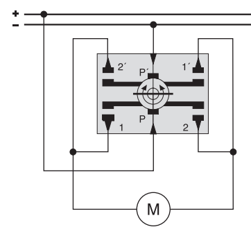
1 Gleichspannungsantrieb
