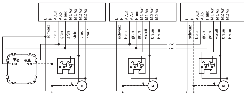
Rollladen-Mehrfachsteuerrelais-Einsätze
