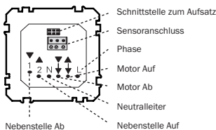
Jalousiesteuerungs-Einsatz mit Nebstelleneingang (Art.-Nr. 580699)
