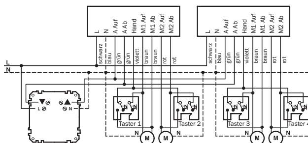
Rollladen-Mehrfachsteuerrelais-Einsätze
