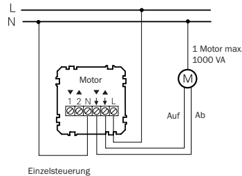
Einzelsteuerung
