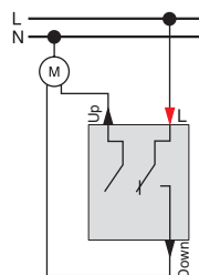
Rollladenschalter, 1-polig MEG3715-0000
