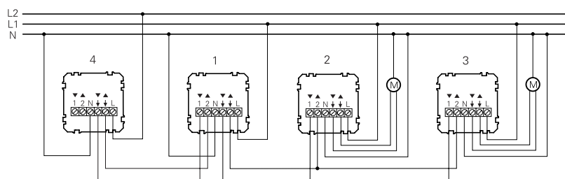
Anschluss von Einsätzen auf unterschiedlichen Phasen
