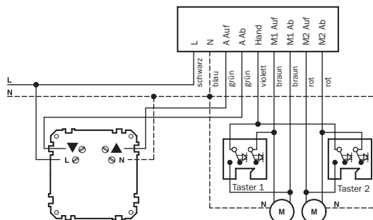
Rollladen-Mehrfachsteuerrelais-Einsatz
