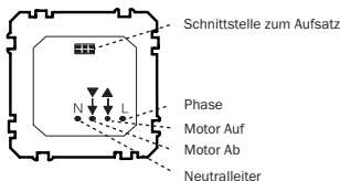
Jalousiesteuerungs-Einsatz Standard (Art.-Nr. 580698)
