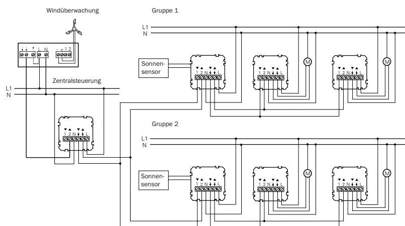
Zentralsteuerung mit Windüberwachung und Gruppensteuerung
