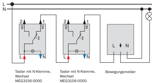
ARGUS in vorhandene Wechselschaltung mit Wechsel-taster als Öffner geschaltet
