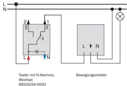
ARGUS mit Wechseltaster als Öffner geschaltet (für Nachinstallation)
