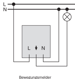
ARGUS ständig am Netz
