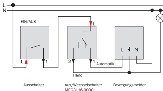
ARGUS geschaltet mit Ausschalter und mit Wechselschalter
