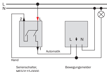
ARGUS geschaltet mit Serienschalter
