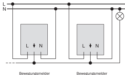
ARGUS ständig am Netz parallel geschaltet
