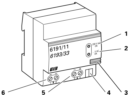
Fig. 1: Geräteabbildung
